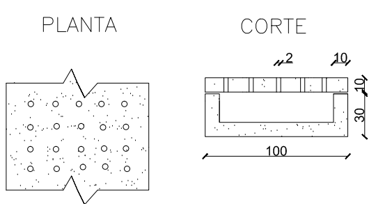
DETALHE 01 – CANALETA EM CONCRETO COM GRELHA EM CONCRETO ARMADO
