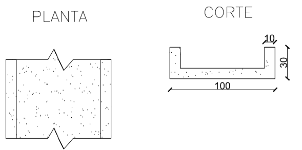
DETALHE 02 – CANALETA EM CONCRETO
