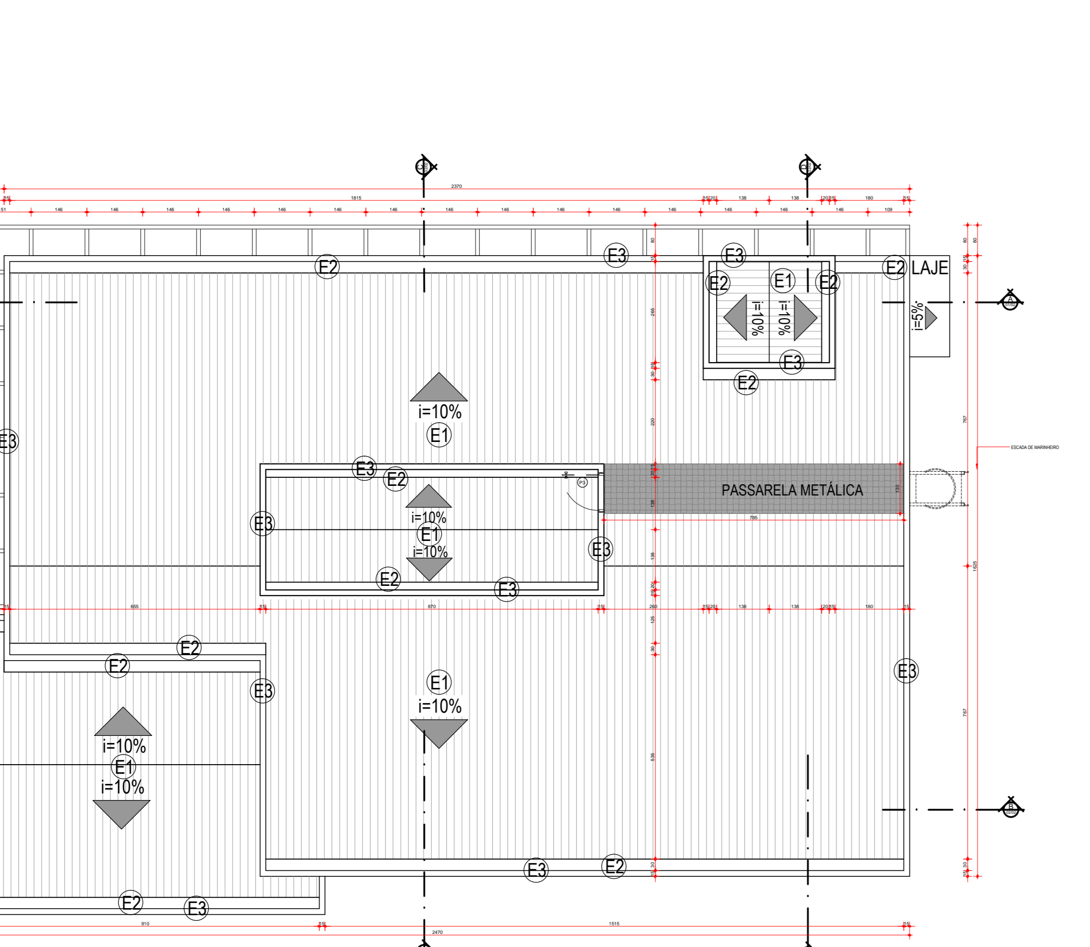
PLANTA DE COBERTURA ESC: 1/100
