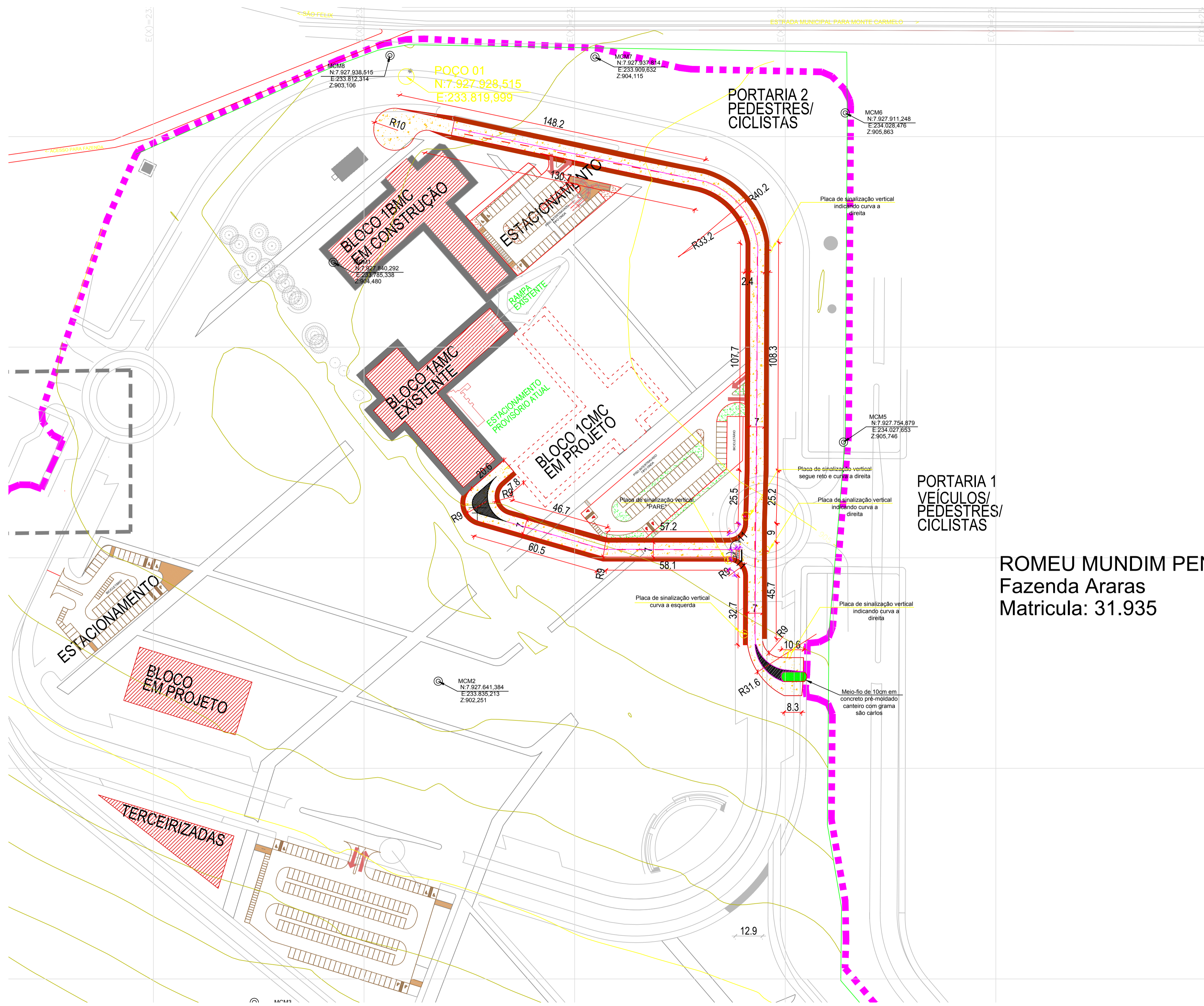
01 TRAÇADO VIÁRIO PROVISÓRIO CAMPUS MONTE CARMELO ESC.: 1/2000
