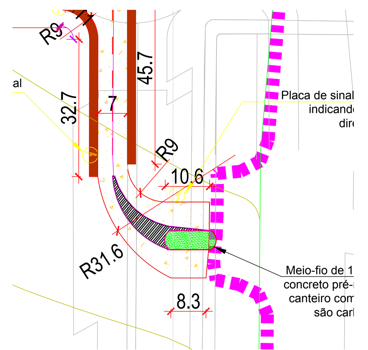
02 DETALHE 01 CAMPUS MONTE CARMELO ESC.: 1/500
