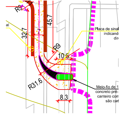
02 DETALHE 01 CAMPUS MONTE CARMELO ESC: 1/500
