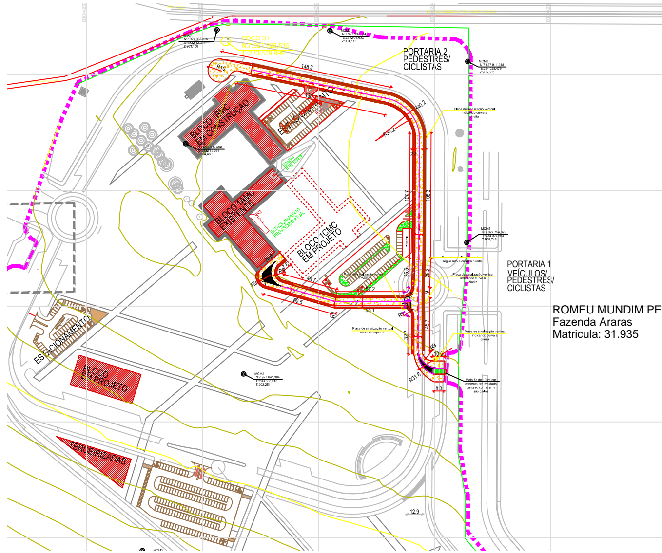
01 TRAÇADO VIÁRIO PROVISÓRIO CAMPUS MONTE CARMELO ESC: 1/2000
